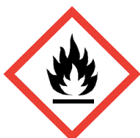
GHS02
